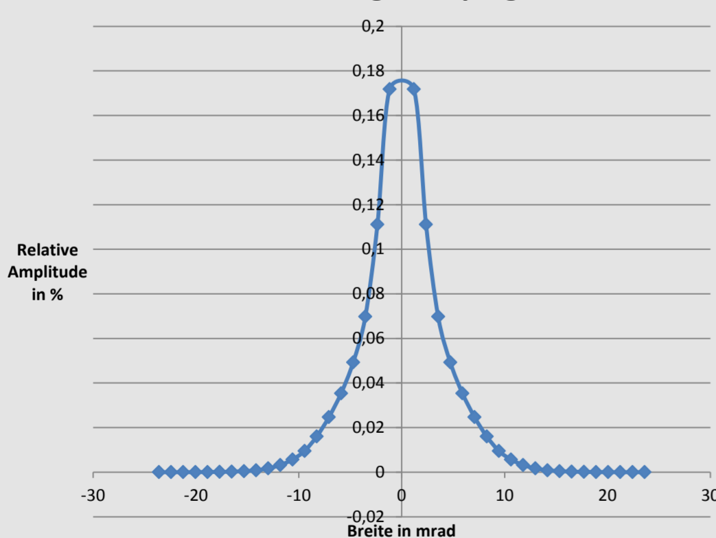
Gauß-Streuung der Spiegel
