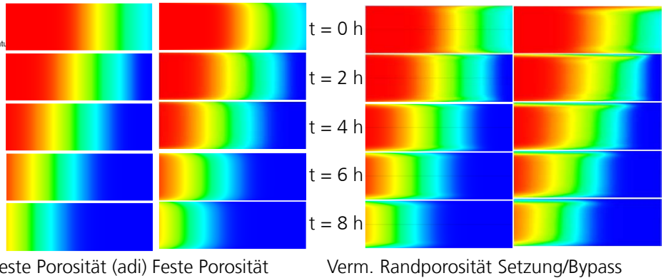
Abbildung 2: Temperaturprofile (Solid) Entladevorgang
