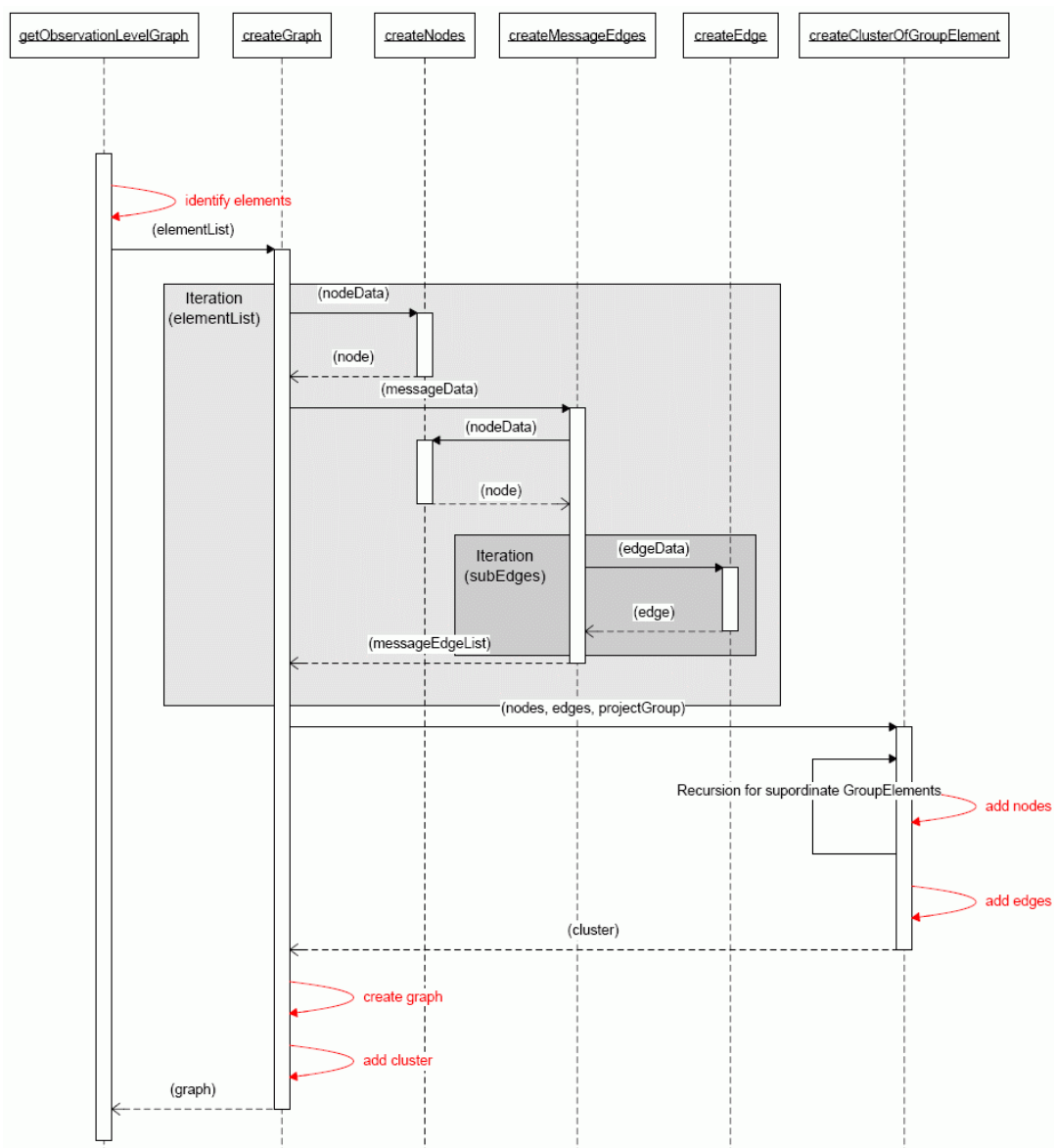
Abbildung 21: Sequenzdiagramm zur Erstellung eines Observationlevelgraphen
