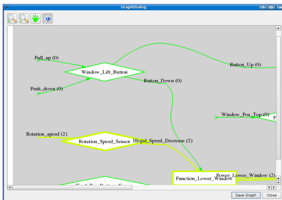
Abbildung 23: Screenshot des GraphDialogs
