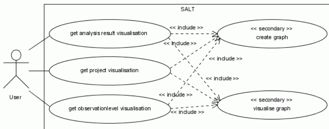
Abbildung 12: Usecasediagramm
