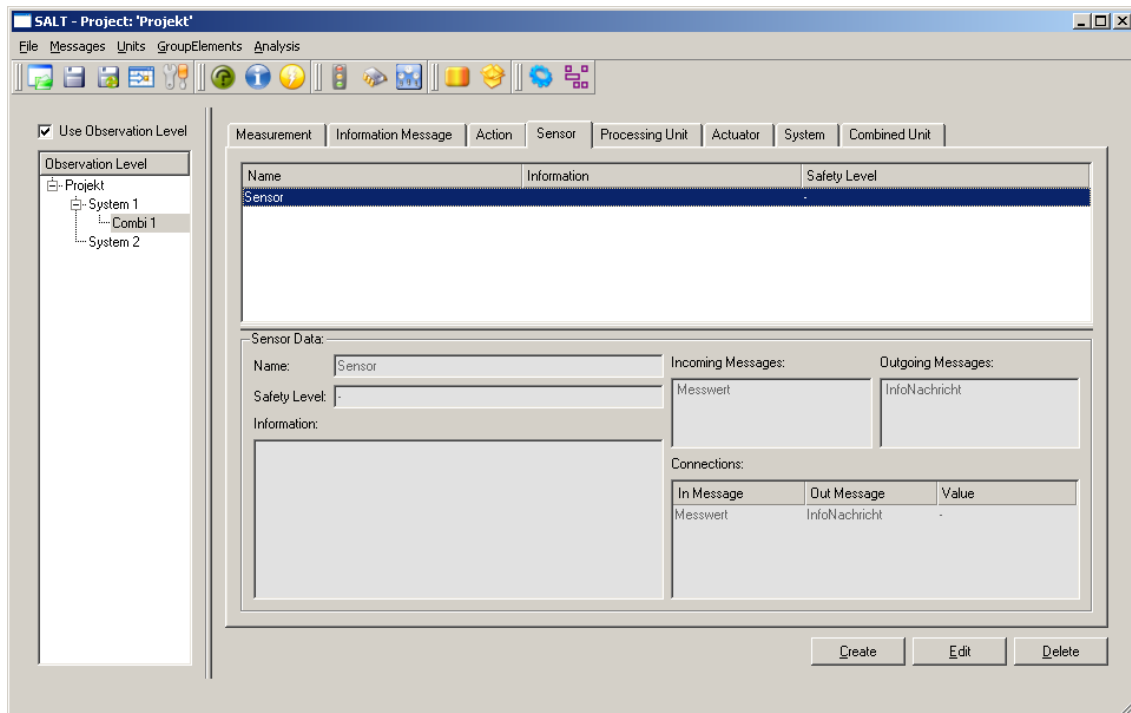
Abbildung 9: Hauptfenster nach Einführung der Observationsschichten
