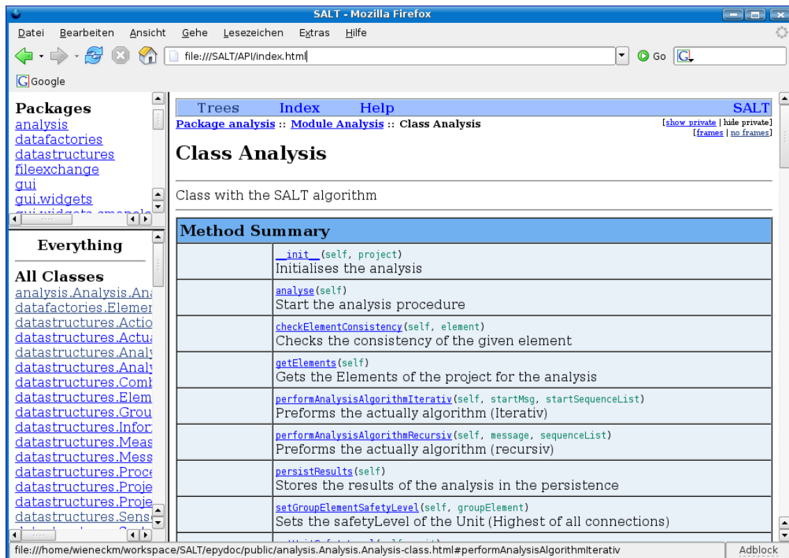
Abbildung 26: SALT-API
