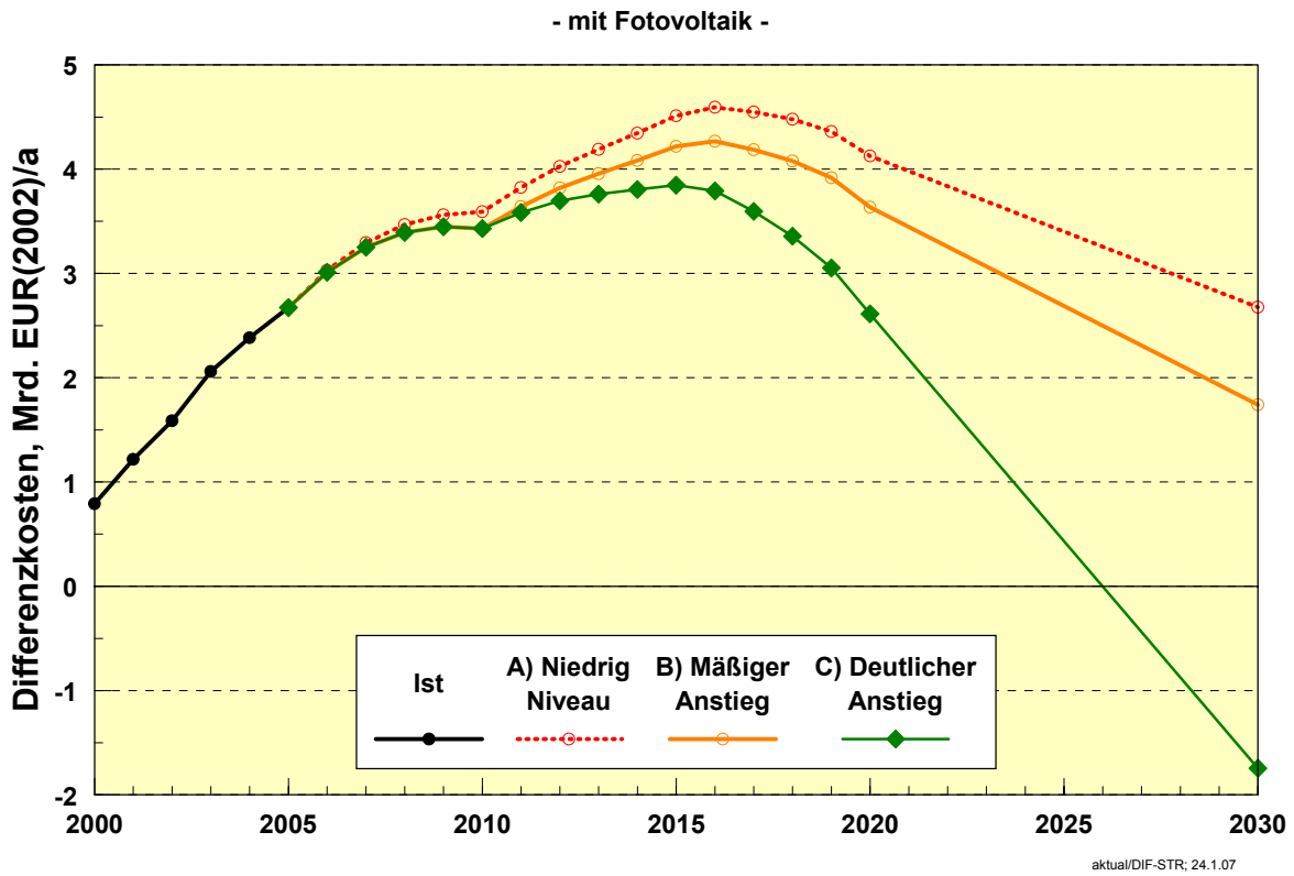
Abbildung 3.18: Gesamte Differenzkosten der EE-Stromversorgung in Abhängigkeit unterschiedlicher Preispfade für fossile Brennstoffe und CO 2 -Preise.
