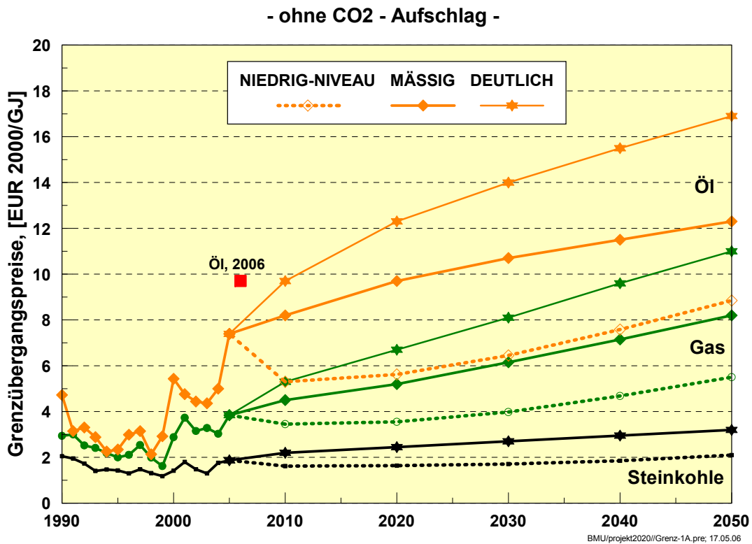
Abbildung 3.8: Grenzübergangpreise für Öl, Erdgas und Steinkohle in allen Preispfaden (ohne CO 2 -Aufschlag). Für Steinkohle sind nur die Pfade A und C eingetragen
