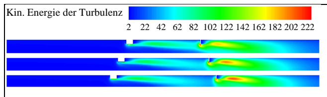
Abbildung 3: Verteilung der kinetischen Energie der Turbulenz k für die Abstände l=300 mm, 400 mm und 500 mm bei einer mittleren Geschwindigkeit von 20 m/s, k - \epsilon Turbulenzmodell mit Wandfunktionen
