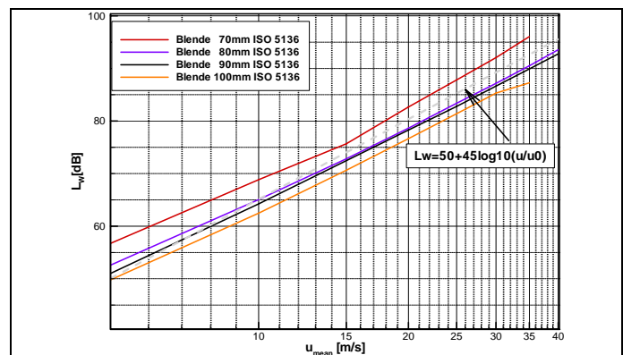
Abbildung 2: Abhängigkeit der Schallleistung durch Blenden mit den Innendurchmessern d_i=70 mm, 80 mm, 90 mm bzw. 100 mm (ohne Blende) von der mittleren Strömungsgeschwindigkeit u_{\text{mean}}
