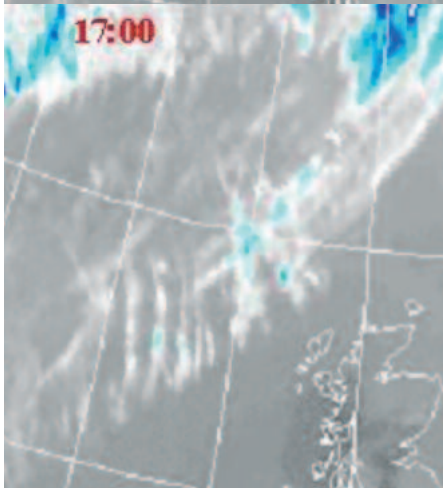
Eine Serie von METEOSAT Infrarot-Kanal-Bildern für die Region des nordatlantischen Flugkorridors nordwestlich Schottlands zeigt Wolken unterschiedlicher Temperatur. Die blaue Farbe charakterisiert Temperaturen unter -40^{\circ}\text{C} . Die Zeiten beziehen sich auf Weltzeit (UTC). Man erkennt den Übergang von Kondensstreifen zu Zirren (H. Mannstein, DLR)
