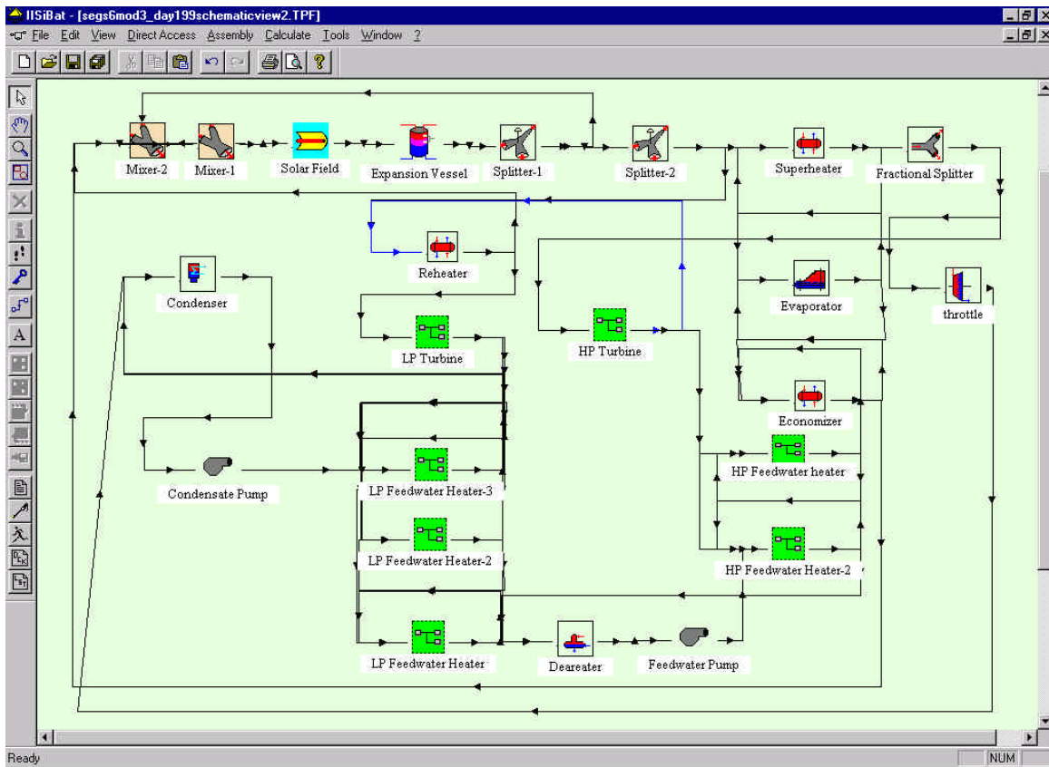
Fig.3. The SEGS VI TRNSYS model.
