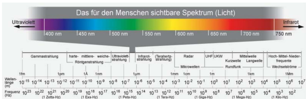
Bild 1: Elektromagnetisches Spektrum
