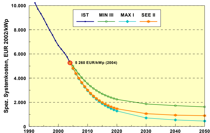
Abb. 4: Entwicklung mittlerer PV-Systemkosten (EUR 2002 /kW p ) in Abhängigkeit der Kombination von Marktwachstum (Szenarien MIN, SEE, MAX) und Lernfaktoren (Fälle I, II, III).
