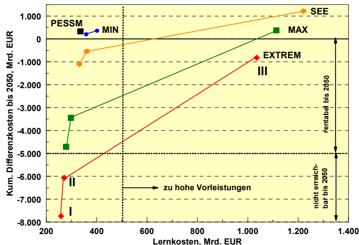
Abb. 5: Kumulierte Differenzkosten (2000-2050) verschiedener PV-Ausbaustrategien in Verknüpfung mit den notwendigen Lernkosten bis zum Break-even Zeitpunkt (Preisvariante „wirksamer“ Klimaschutz) für die Lernkurvenfälle I (jeweils linke Datenpunkte) bis III (jeweils rechte Datenpunkte)
