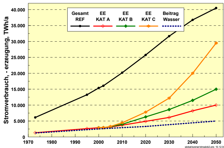
Abb. 1: Korridor des Beitrags erneuerbarer Energien (Szenarienkategorien A, B und C) an der globalen Stromversorgung bis 2050 (Referenzentwicklung) und Berücksichtigung des noch möglichen Beitrags der Wasserkraft.
