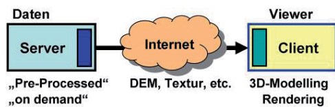
Abbildung 3 Systemaufbau der Echtzeitvisualisierung für „clientseitiges Rendering“
