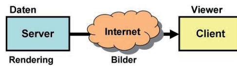
Abbildung 2 Systemaufbau der Echtzeitvisualisierung für „serverseitiges Rendering“
