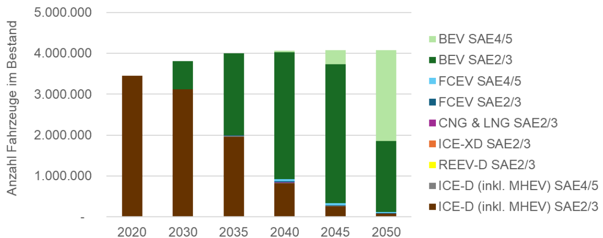
Abbildung 41: Entwicklung der simulierten Bestands-Marktanteile für leichte und schwere Nutzfahrzeuge im Alternativszenario Automatisierung
