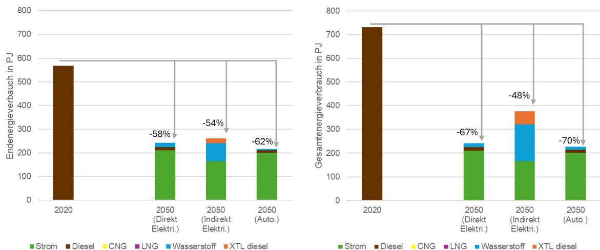
Abbildung 48: Endenergieverbrauch und Gesamtenergieverbrauch des Straßenverkehrs im 2050 im Vergleich je Szenario
