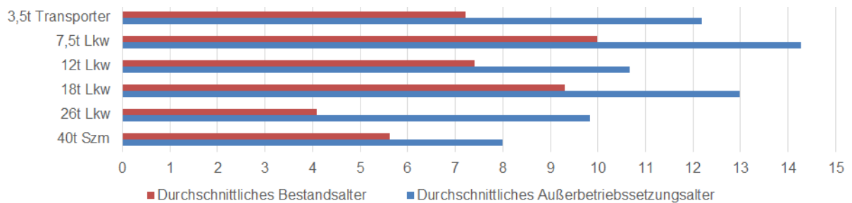
Abbildung 6: Durchschnittliches Bestandsalter und bereinigte Außerbetriebssetzungsalter nach Fahrzeugsegment (eigene Darstellung in Anlehnung an [59])
