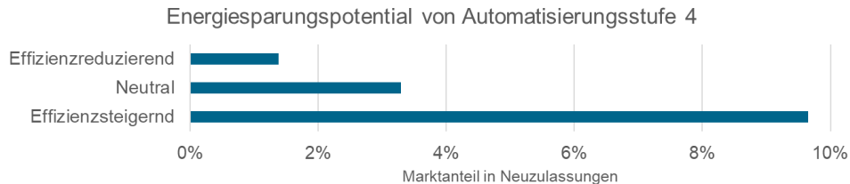
Abbildung 29: Veränderung des Marktpotenzials von Fahrzeugkonzepten mit Automatisierungsstufe 4 im Segment 40 t Sattelzugmaschinen im Fernverkehr unter verschiedenen Annahmen zur Energieeffizienzwirkung
