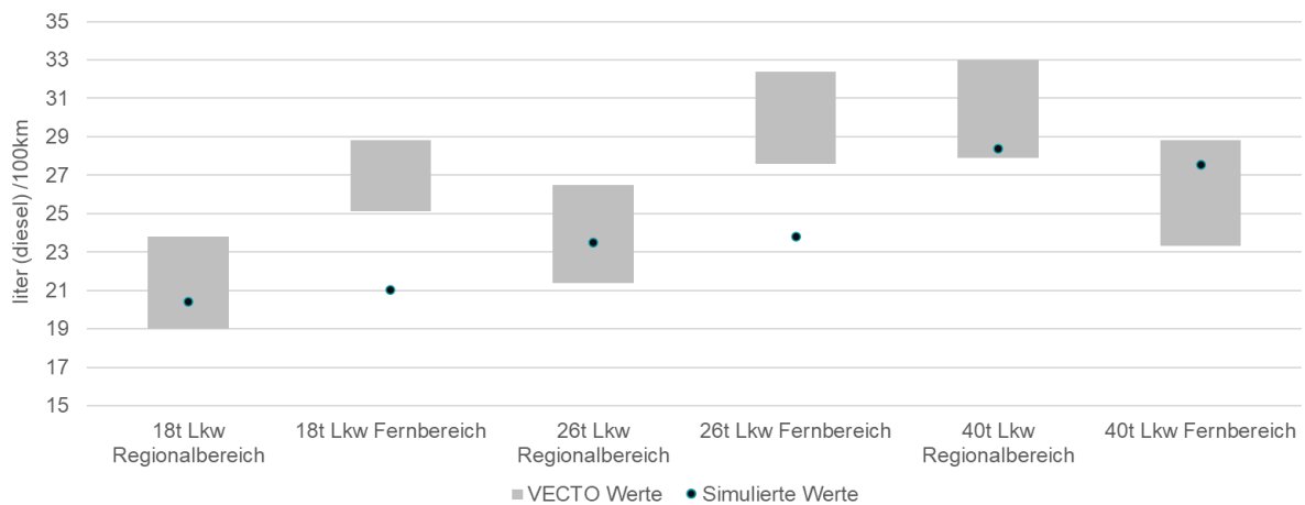
Abbildung 31: Vergleich der simulierten und VECTO-basierten Energieverbräuche schwerer Dieselnutzfahrzeuge in Deutschland
