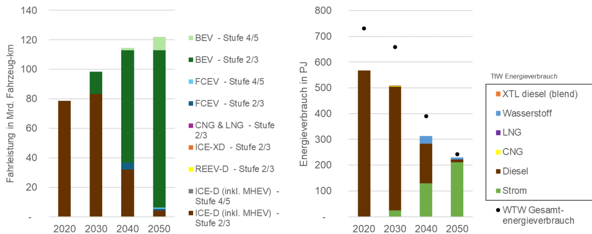
Abbildung 42: Entwicklung der Fahrleistung (links) und des Endenergieverbrauchs (rechts) im Straßengüterkraftverkehr in Deutschland bis 2050 im Referenzszenario „Direkte Elektrifizierung“
