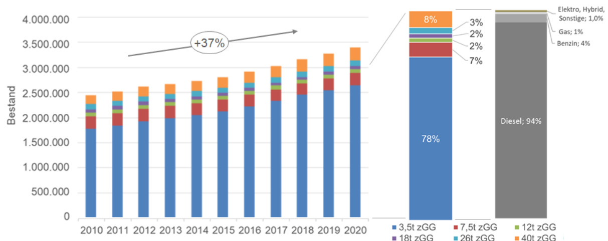
Abbildung 4: Entwicklung des jährlichen Fahrzeugbestands im deutschen Straßengüterkraftverkehr nach Fahrzeugsegmenten (eigene Auswertung in Anlehnung an [57])
