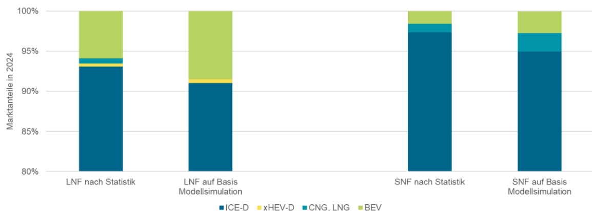
Abbildung 32: Vergleich modellierter und statistisch erfasster Marktanteile konventioneller und alternativer Antriebskonzepte im Jahr 2024
