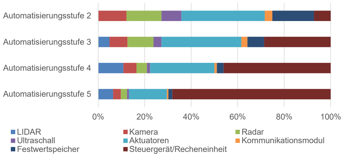
Abbildung 17: Verteilung des fahrzeuginternen Energiebedarfs der Automatisierungssysteme nach Komponenten und Automatisierungsstufe
