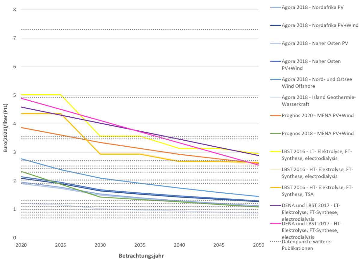
Abbildung 54: Literaturübersicht prognostizierter PtL-Gestehungskosten für großskalige Produktionskapazitäten (auf Basis [99–106])
