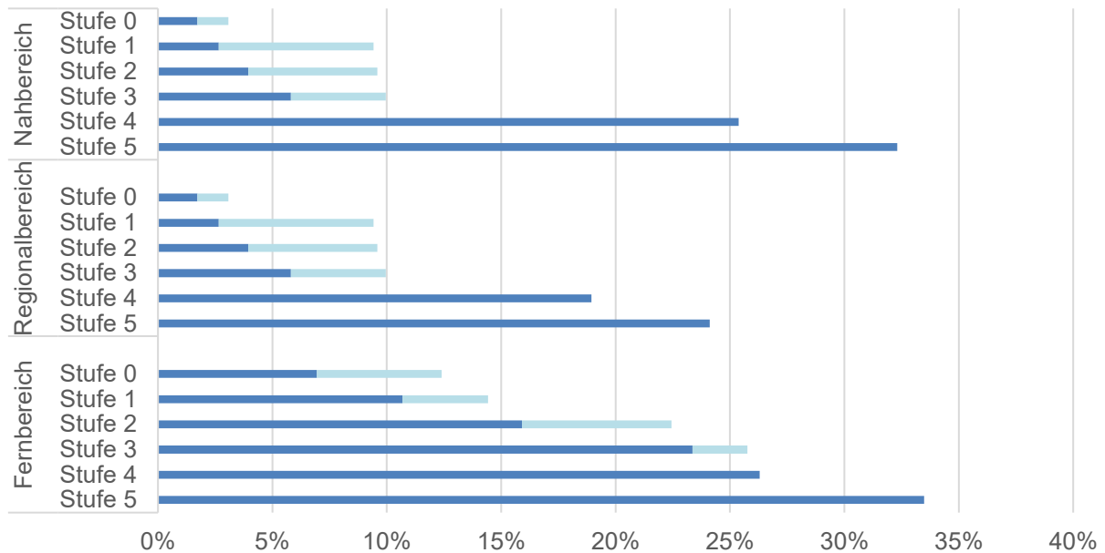
Abbildung 21: Berechnetes Sicherheitspotential je Automatisierungsstufe und Einsatzbereich (dunkle Balken stellen die Mindestpotentiale da, helle Balken die Maximalpotentiale)
