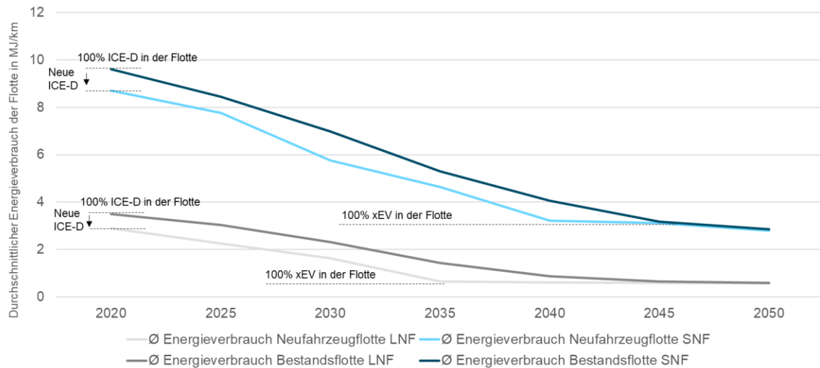
Abbildung 43: Entwicklung des durchschnittlichen Energieverbrauchs der Neu- und Bestandsfahrzeugflotte jeweils für leichte (LNF) und schwere Nutzfahrzeuge (SNF) im Referenzszenario „direkte Elektrifizierung“
