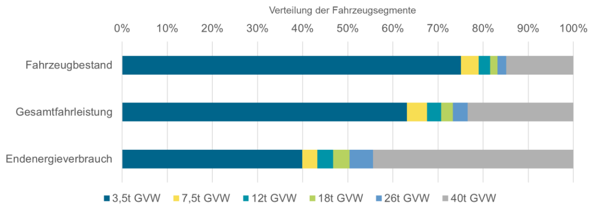
Abbildung 30: Verteilung des Fahrzeugbestands, der Gesamtfahrleistung und des Endenergieverbrauchs nach Fahrzeugsegmenten im Jahr 2030
