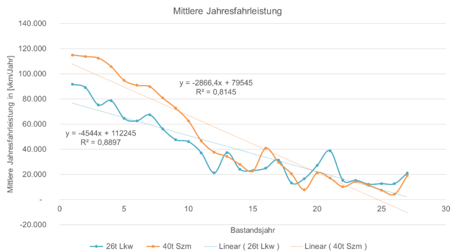
Abbildung 53: Entwicklung der mittlere Jahresfahrleistung in Abhängigkeit ihres Fahrzeugalters (eigene Darstellung in Anlehnung an [60])
