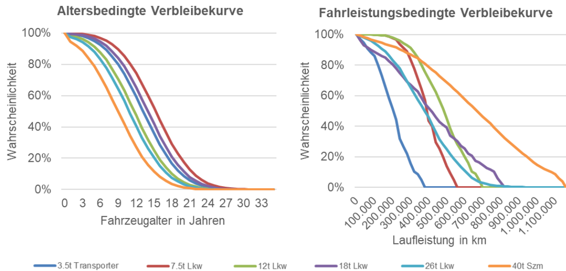
Abbildung 26: Alters- und fahrleistungsbedingte Verbleibekurve je Nutzfahrzeugsegment
