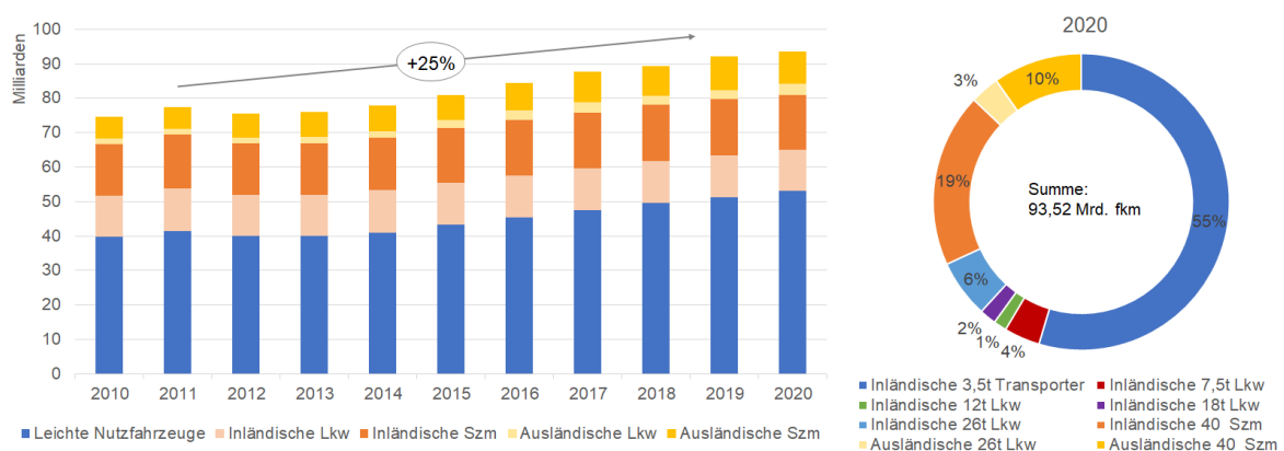
Abbildung 7: Entwicklung der Inlandsfahrleistung (in FzKm) des Straßengüterkraftverkehrs (in Anlehnung an [49, 50, 61])
