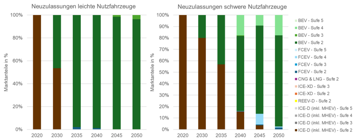
Abbildung 33: Entwicklung der simulierten Neuzulassungen-Marktanteile für leichte (linke Abbildung) und schwere (rechte Abbildung) Nutzfahrzeuge im Referenzszenario direkte Elektrifizierung
