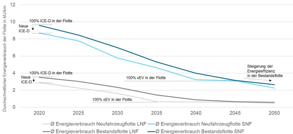
Abbildung 47: Entwicklung des durchschnittlichen Energieverbrauchs der Neu- und Bestandsfahrzeugflotte jeweils für leichte (LNF) und schwere Nutzfahrzeuge (SNF) im Alternativszenario „Automatisierung“
