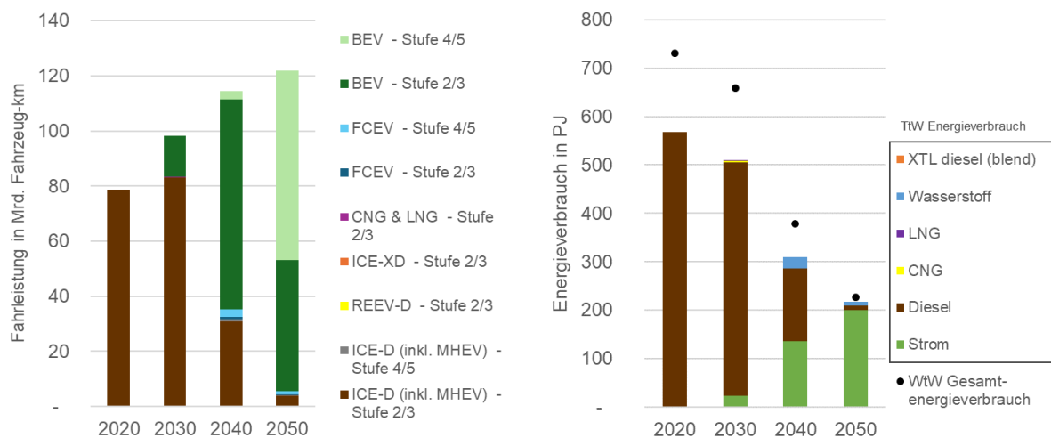
Abbildung 46: Entwicklung Fahrleistung (links) und Endenergieverbrauch (rechts) Straßengüterkraftverkehr in Deutschland bis 2050 Alternativszenario „Automatisierung“
