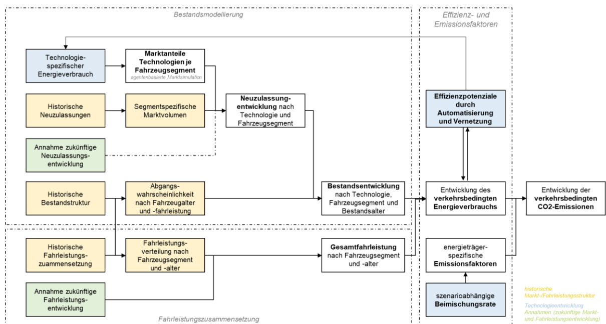
Abbildung 25: Schematische Darstellung zur Berechnung der verkehrsbedingten CO 2 -Emissionen unter Berücksichtigung alternativer Fahrzeugtechnologien und Kraftstoffe (Konzeptionelles Modell)
