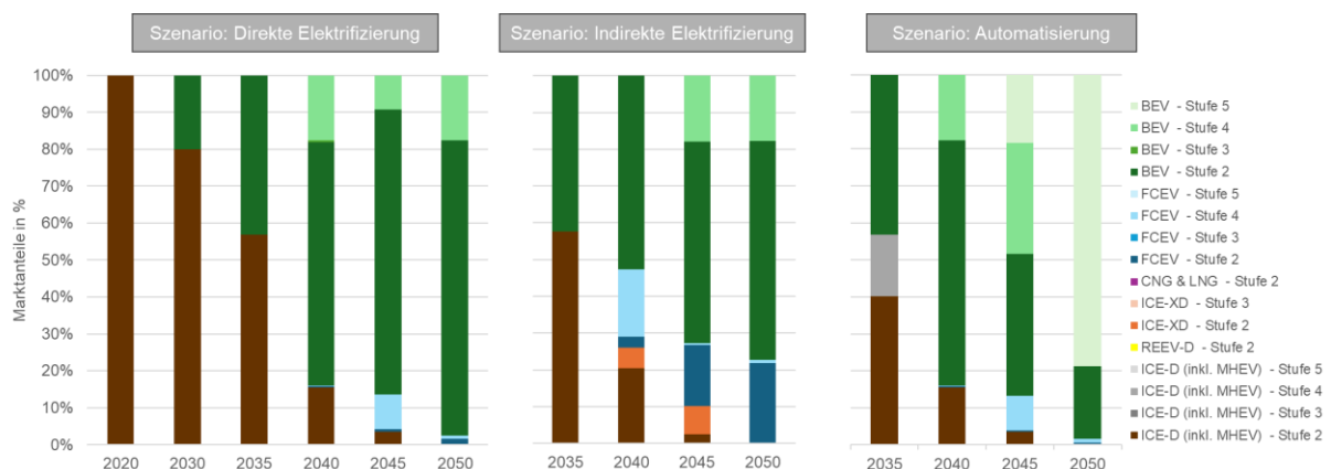
Abbildung 49: Vergleich der Marktpotentiale konkurrierender Antriebsstrang- und Automatisierungstechnologien im schweren Nutzfahrzeugmarkt in verschiedenen Szenarien
