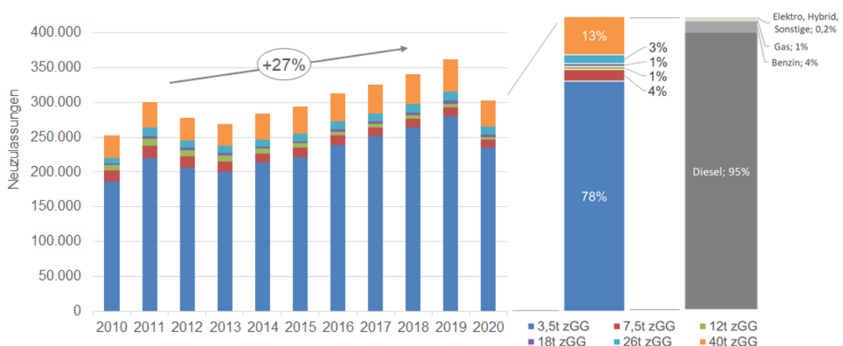
Abbildung 3: Entwicklung der jährlichen Neuzulassungen im deutschen Straßengüterkraftverkehr nach Fahrzeugsegmenten (eigene Auswertung in Anlehnung an [59])
