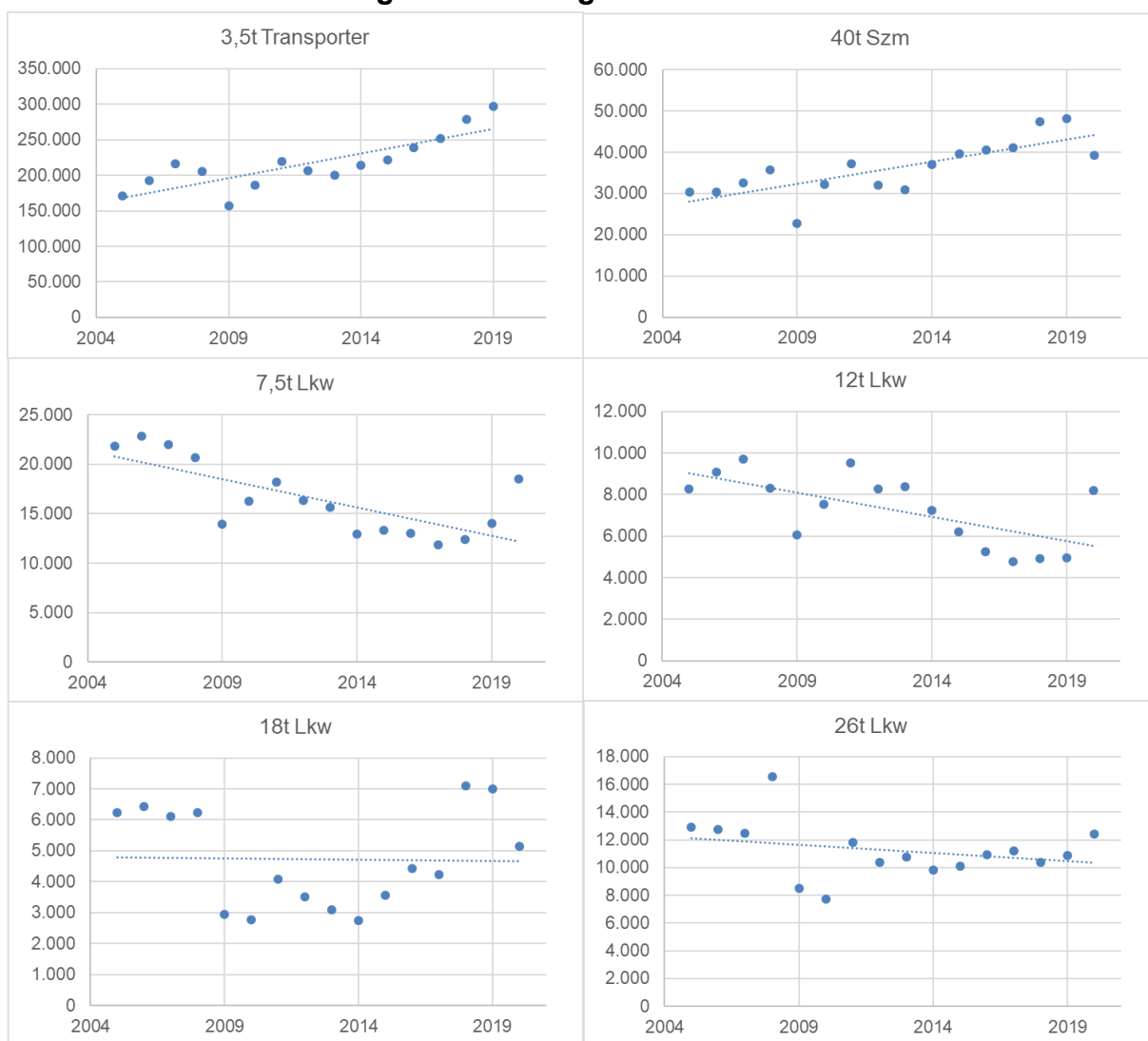
Abbildung 51: Entwicklung der segmentspezifischen Neuzulassungen zwischen 2005 und 2020 (X-Achse: Jahre, Y-Achse: Neuzulassungen) (eigene Darstellung in Anlehnung an [57, 59])
