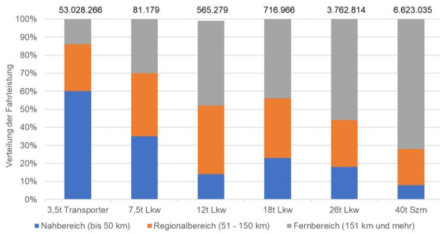
Abbildung 10: Segmentspezifische Verteilung der Fahrleistung nach Einsatzbereiche mit Angabe der absoluten Fahrleistung in 1.000 km (eigene Darstellung in Anlehnung an [61])
