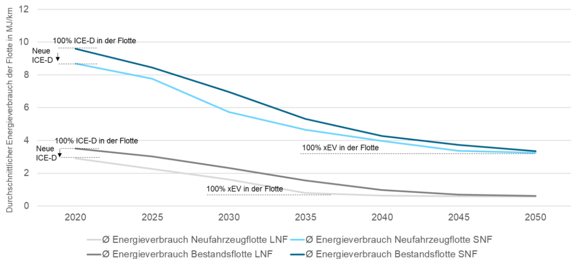
Abbildung 45: Entwicklung des durchschnittlichen Energieverbrauchs der Neu- und Bestandsfahrzeugflotte jeweils für leichte (LNF) und schwere Nutzfahrzeuge (SNF) im Alternativszenario „indirekte Elektrifizierung“
