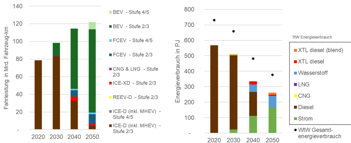
Abbildung 44: Entwicklung der Fahrleistung (links) und des Endenergieverbrauchs (rechts) im Straßengüterkraftverkehr in Deutschland bis 2050 im Alternativszenario „indirekte Elektrifizierung“
