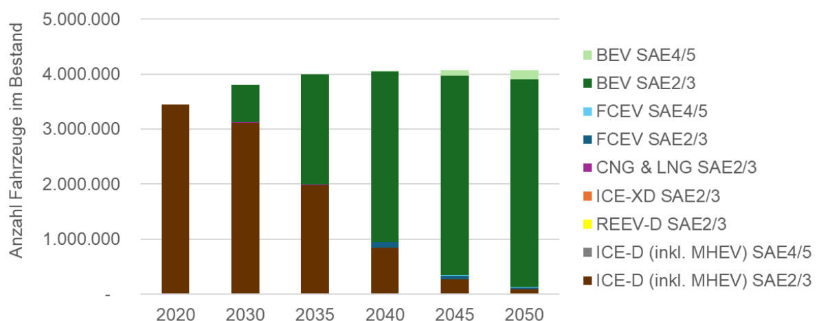
Abbildung 35: Entwicklung der simulierten Bestands-Marktanteile für leichte und schwere Nutzfahrzeuge im Referenzszenario direkte Elektrifizierung
