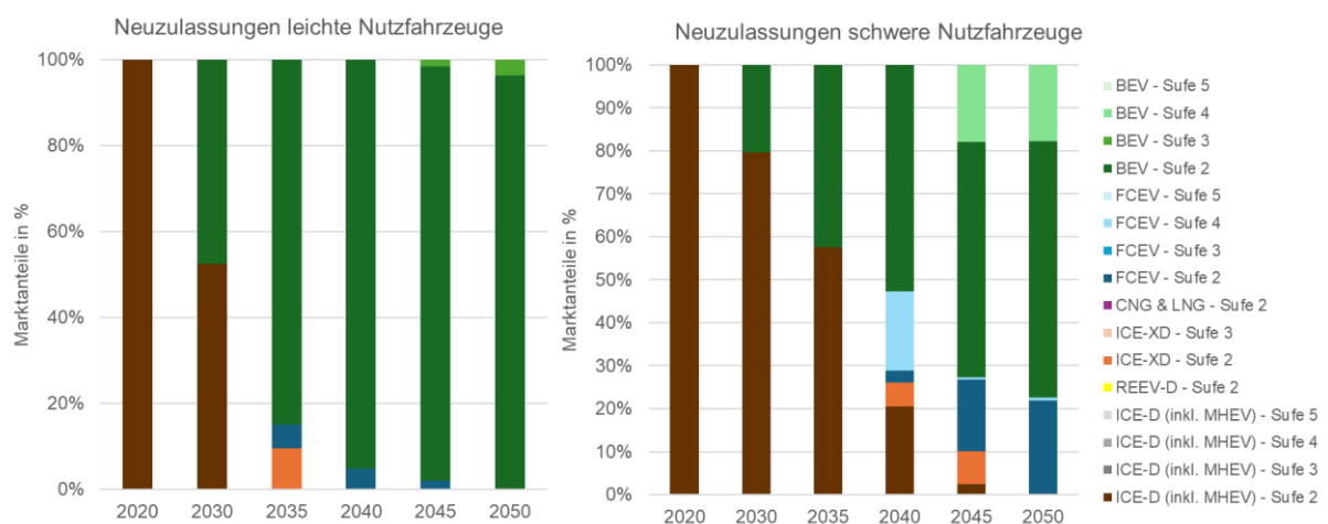
Abbildung 36: Entwicklung der simulierten Neuzulassungen-Marktanteile für leichte (linke Abbildung) und schwere (rechte Abbildung) Nutzfahrzeuge im Alternativszenario indirekte Elektrifizierung
