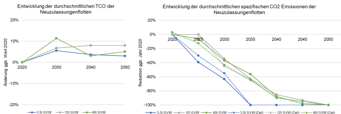
Abbildung 34: Entwicklung der durchschnittlichen Gesamtbetriebskosten (TCO) und spezifischen CO 2 -Emissionen der Neuzulassungsflotten im Referenzszenario direkte Elektrifizierung
