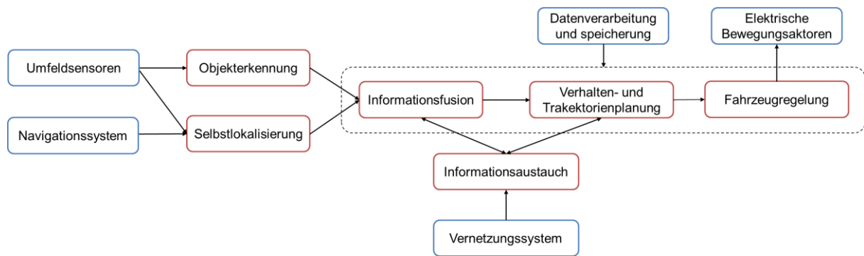
Abbildung 12: Funktionale Architektur automatisierter und vernetzter Fahrzeuge (Eigene Darstellung in Anlehnung an [185])
