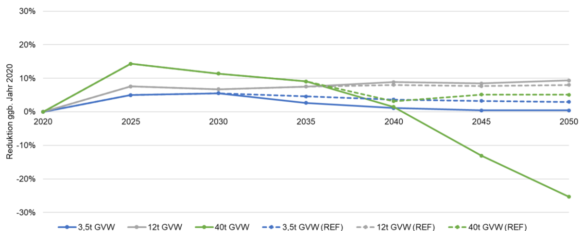
Abbildung 40: Entwicklung der durchschnittlichen Gesamtbetriebskosten (TCO) der Neuzulassungsflotten im Alternativszenario Automatisierung im Vergleich zum Referenzszenario (REF)
