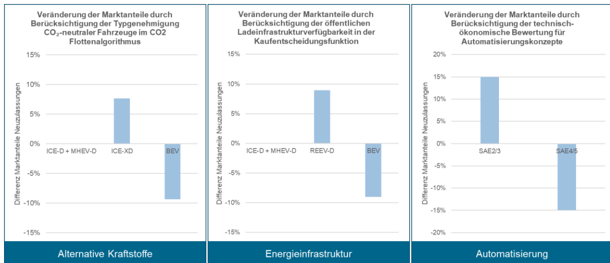
Abbildung 28: Veränderung der Neuzulassung-Marktanteile durch Berücksichtigung alternativer Kraftstoffe, Energieinfrastruktur und Automatisierung gegenüber dem Referenzfall ohne entsprechende Berücksichtigung
