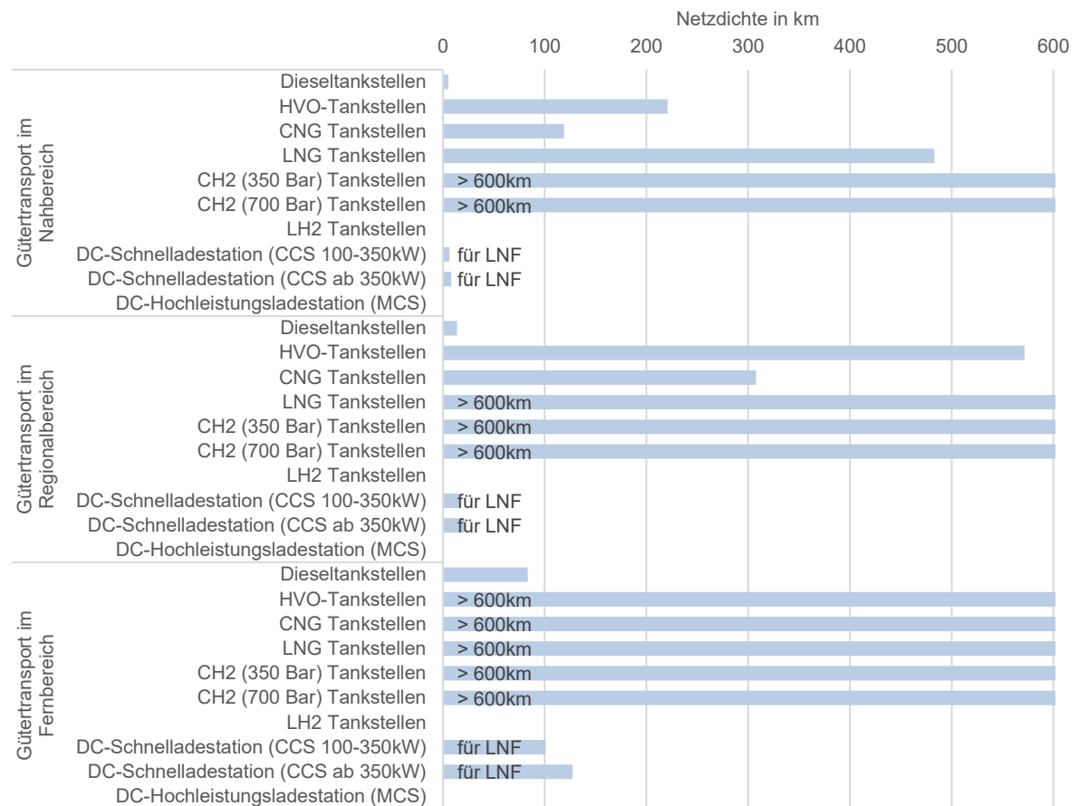
Abbildung 55: Auswertung der Energieinfrastrukturnetzdichte in Deutschland im Jahr 2024 nach Energieträger und Einsatzbereich ([136, 286, 307] sowie Marktdaten aus gas-h2.de, h2-live, h2-mobility.de und bundesnetzagentur.de)
