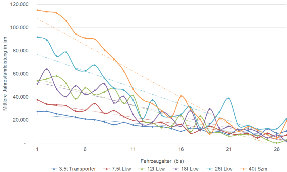
Abbildung 9: Häufigkeitsverteilung der Jahresfahrleistung für einzelne Fahrzeugsegmente in Abhängigkeit ihres Fahrzeugalters (eigene Darstellung in Anlehnung an [60])
