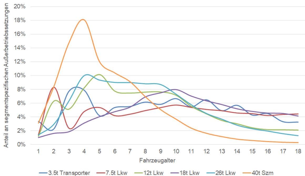
Abbildung 52: Häufigkeitsverteilung der Außerbetriebssetzung nach Fahrzeugsegmente und Fahrzeugalter (In Anlehnung an [59])
