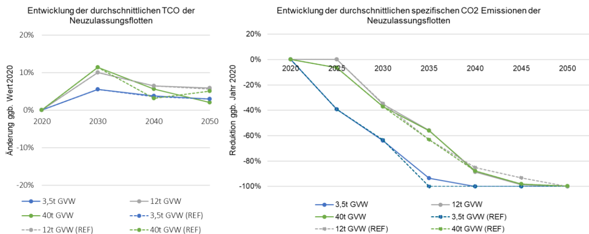
Abbildung 37: Entwicklung der durchschnittlichen Gesamtbetriebskosten (TCO) und spezifischen CO 2 -Emissionen der Neuzulassungsflotten im Alternativszenario indirekte Elektrifizierung im Vergleich zum Referenzszenario (REF)
