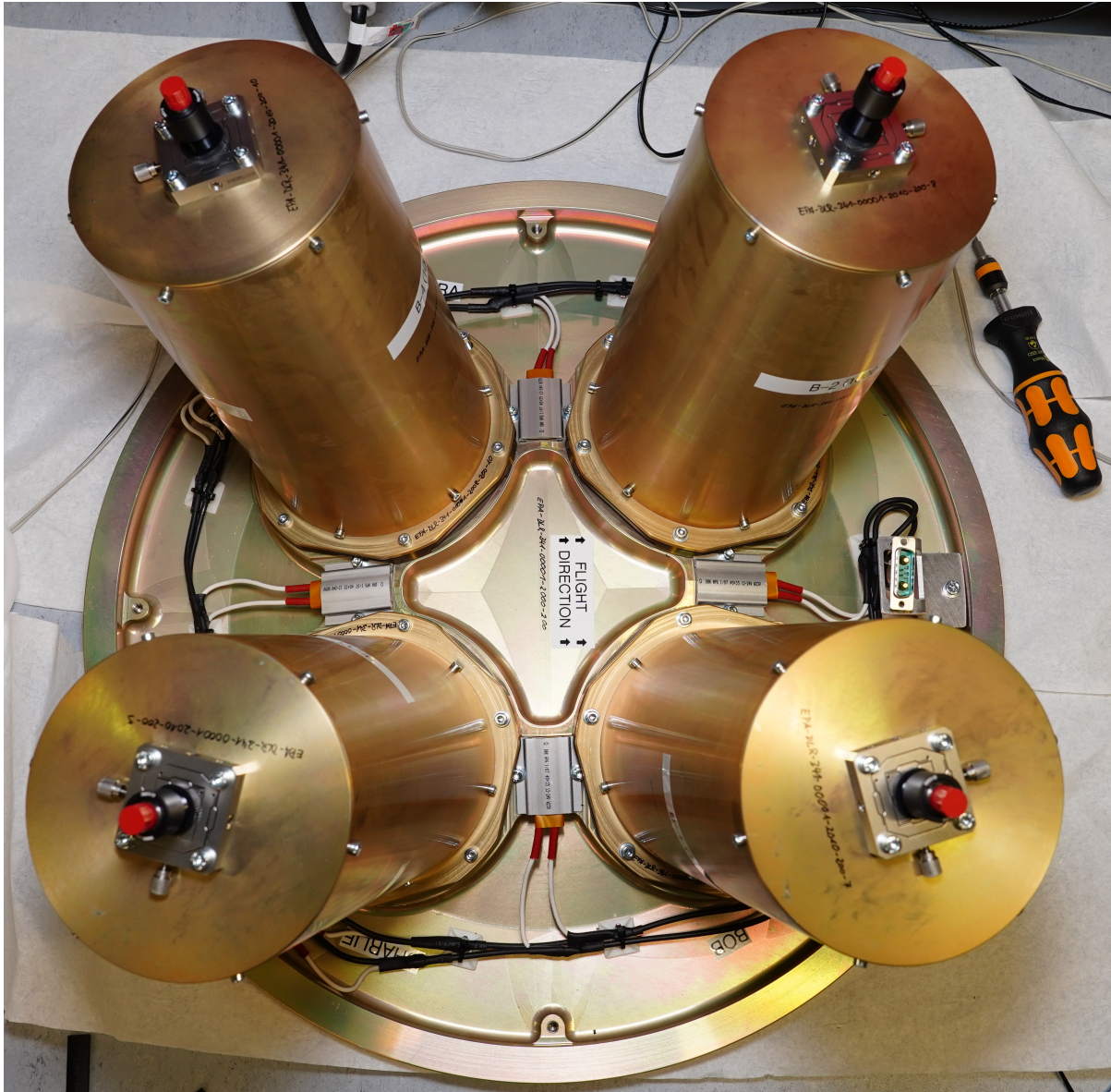
Abbildung 2.7: Montierte Optiken im Labor, die goldfarbenen Tuben ragen später in den Innenraum des Flugzeug. Zwischen den Optiken sind die Heizer angebracht [22].
