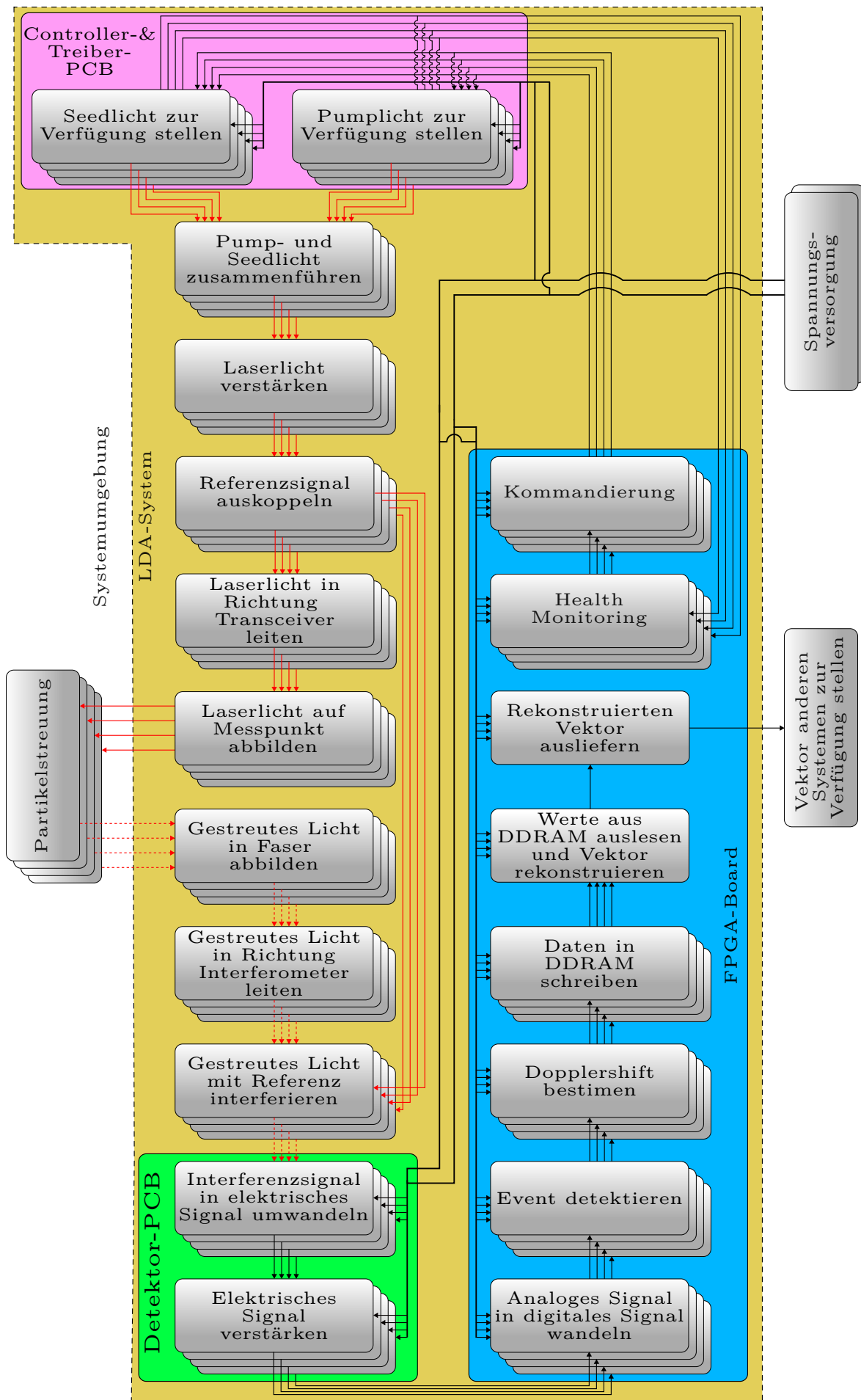
42 Abbildung 5.2: Funktionsblockschartbild über die erforderlichen Systemfunktionen
