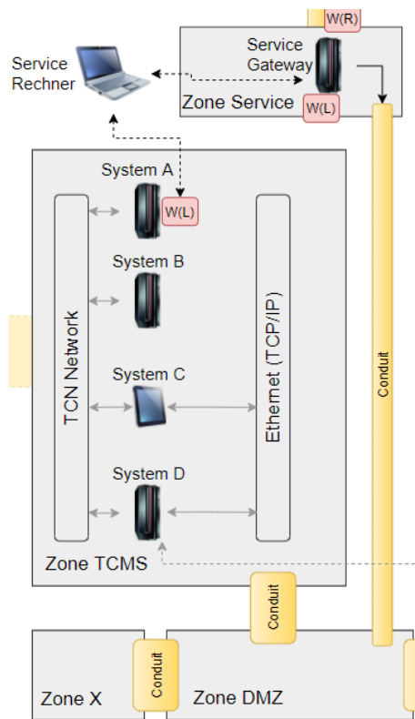
Abbildung 7: Detaildarstellung Zone Fahrzeugtechnik
