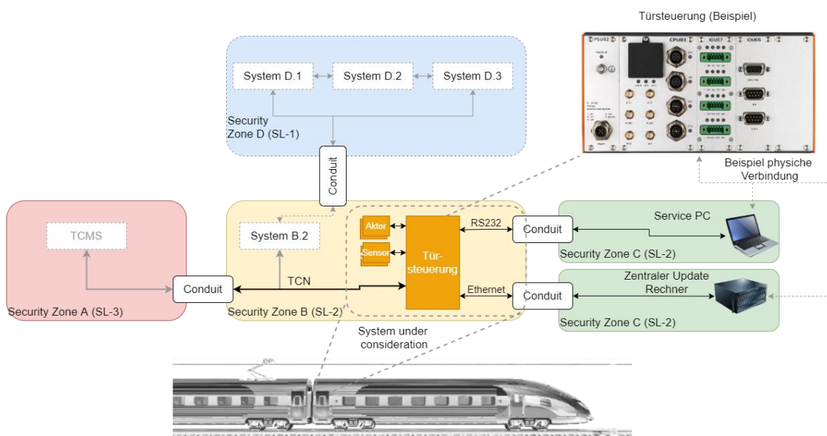
Abbildung 4: Kontext des "System under Consideration" – Türsteuerung
