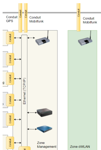
Abbildung 11: Detaildarstellung Security-Zone Fahrgastfunktionen
