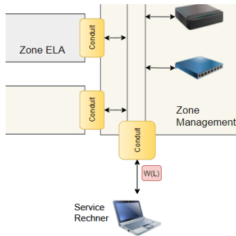
Abbildung 10: Detaildarstellung Management Zugang
