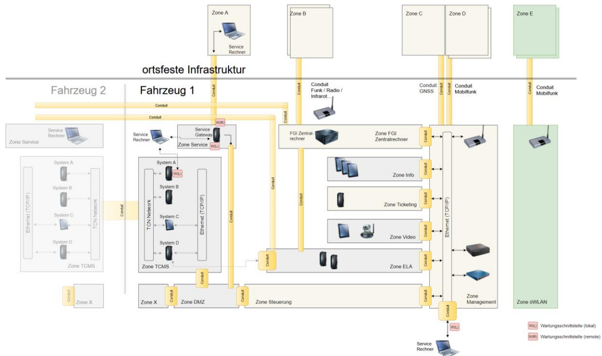
Abbildung 6: Kommunikationsstruktur und IT-Security Zonen einer verallgemeinerten Straßenbahn
