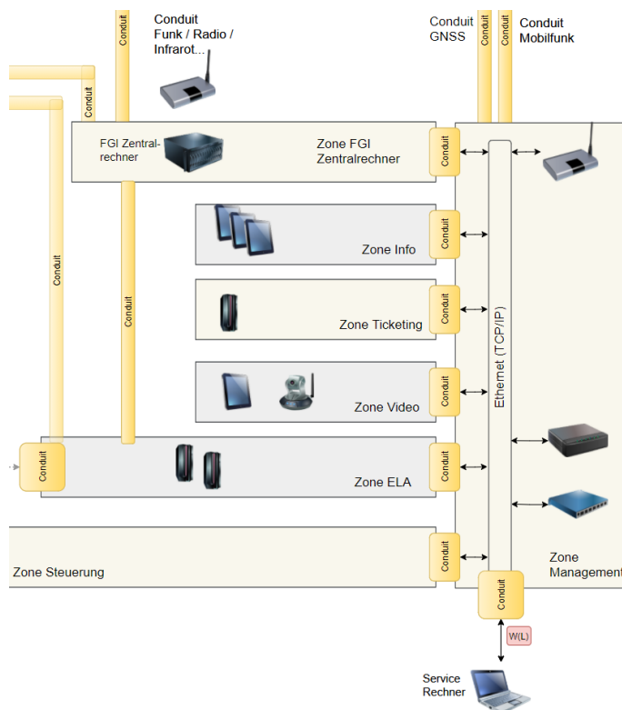
Abbildung 8: Detaildarstellung Security-Zone Betreiber
