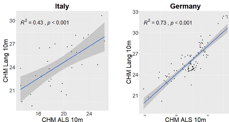
Fig. 5. Validation of the GEDI CHM Lang10m with local ALS CHM LiDAR data at 10 m spatial resolution.
