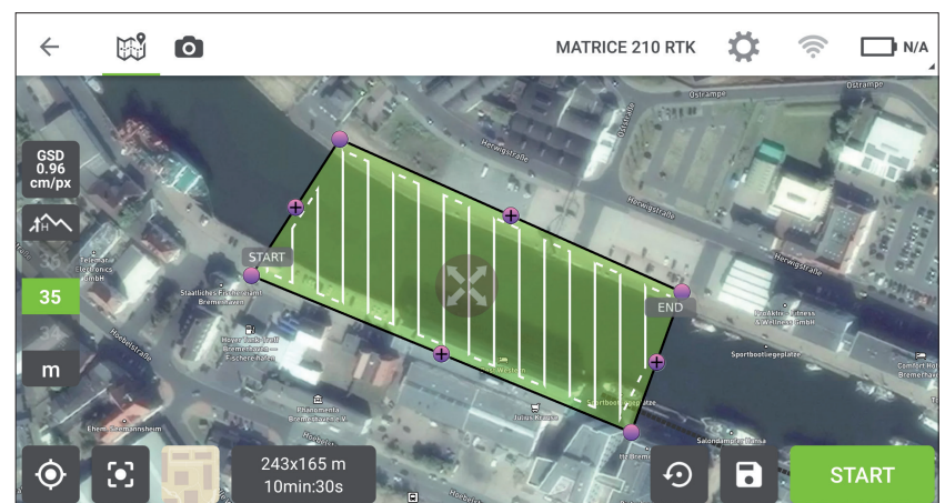
Abb. 1: Planung der Trajektorien des Multikopters mit der Software Pix4Dcapture
