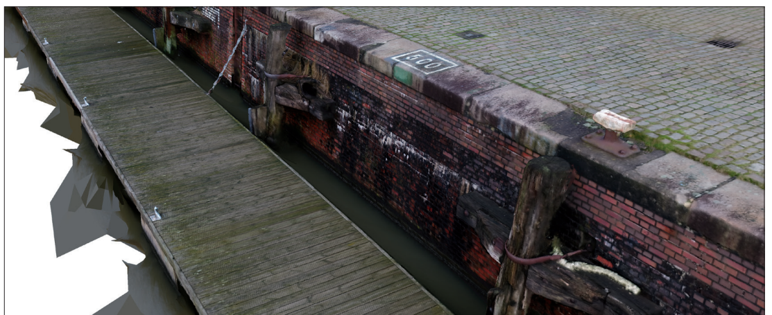
Abb. 3: Ergebnis einer Kaimauerinspektion mit Überflügen in drei unterschiedlichen Höhen, dargestellt mit RealityCapture
