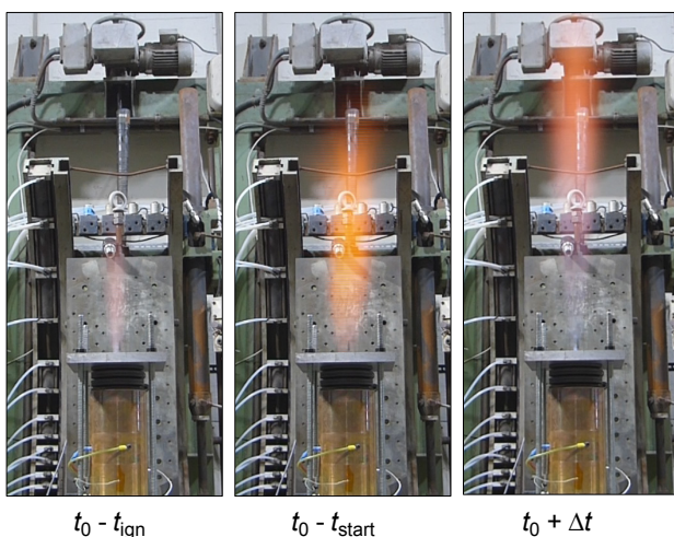
BILD 8. Vor- und Hauptsequenz eines Heißgastests unter Verwendung der Testbrennkammer
