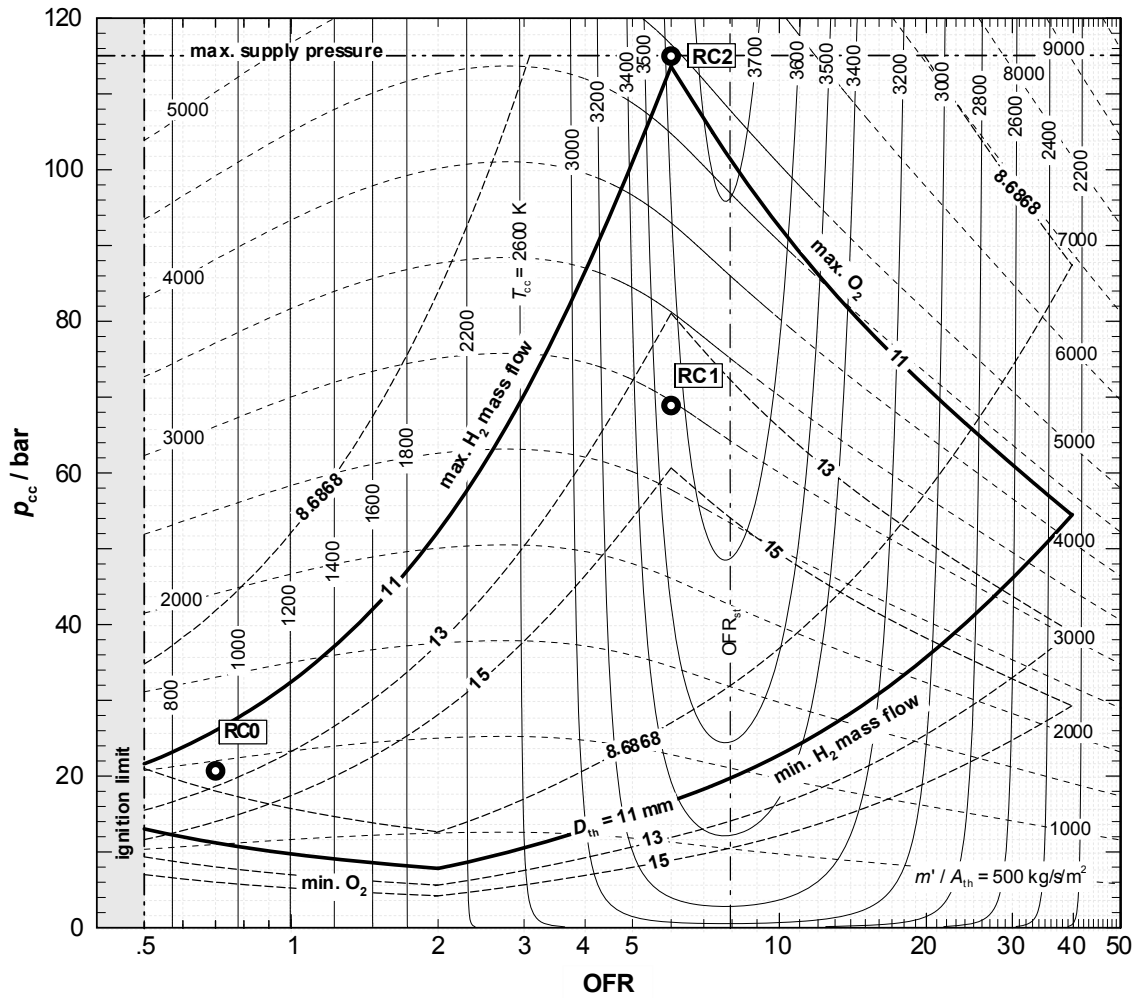
BILD 4. Betriebsbereich der H 2 /O 2 Versorgungsanlage in Abhängigkeit unterschiedlicher Düsenhalsdurchmesser
