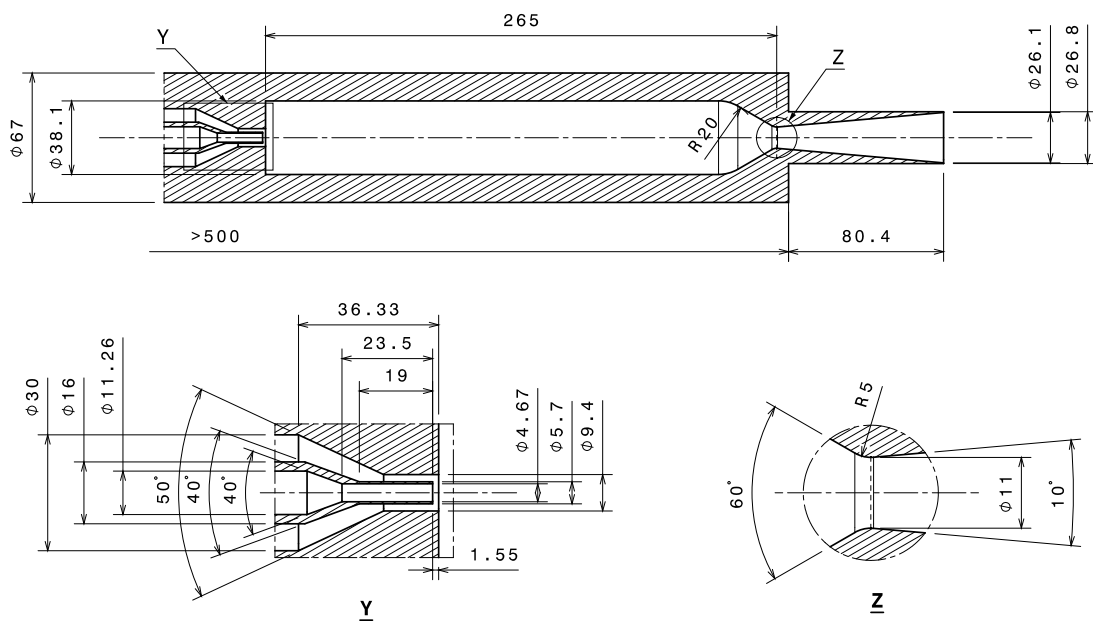
BILD 5. Übersichtsskizze der Außen- und Innengeometrie des Windkanalmodells mit H 2 /O 2 Brennkammer
