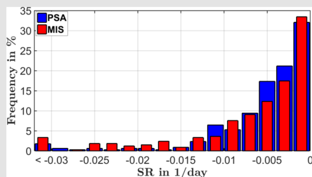
Abbildung 2: Histogramm der mit TraCS auf der PSA und in Missouri gemessenen Soiling-Raten eines Jahres. Im letzten Bin sind alle \xi < -0,03 /Tag zusammengefasst.
