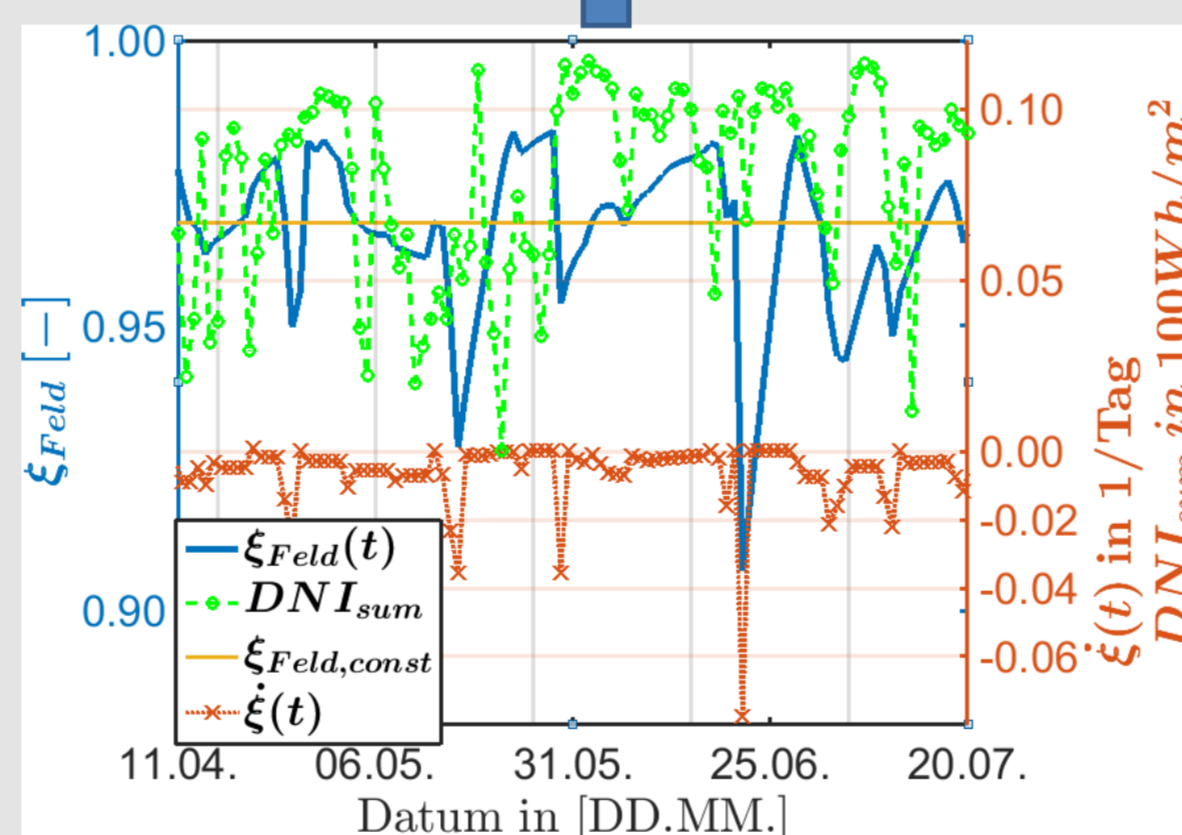
Abbildung 3: Aus \xi(t) und der Reinigungsaktivität berechnete zeitabhängige \xi_{Feld} für die Strategie „Konstant“ mit einem Reinigungsfahrzeug in blau. Jahresmittelwert \xi_{Feld, const} = \text{mean}(\xi_{Feld}(t)) in gelb. Die mit \xi_{Feld} multiplizierten Stundenwerte der DNI werden als Input für greenius verwendet.
