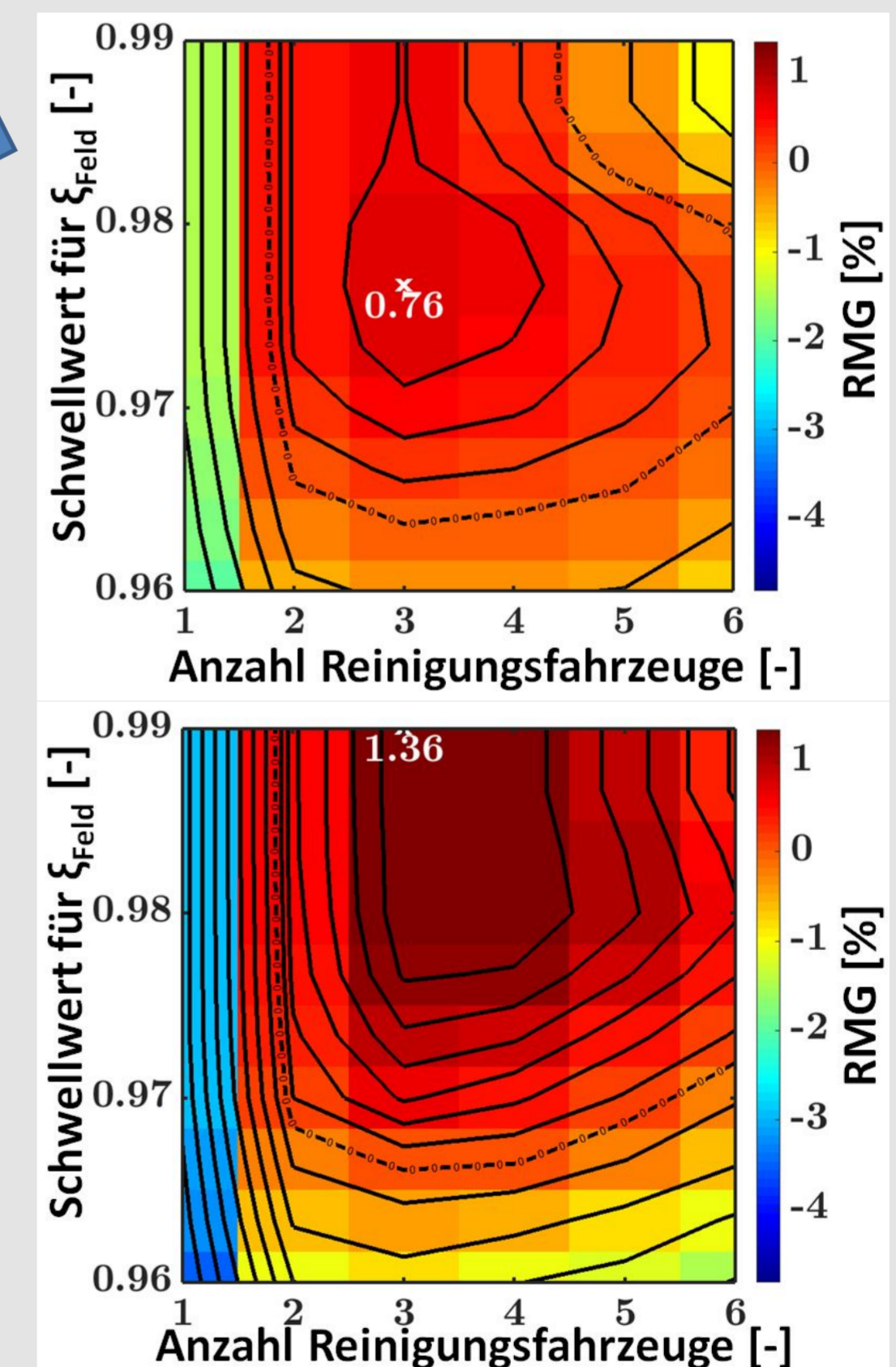
Abbildung 4: relativer Mehrertrag im Vergleich zur Referenzstrategie (RMG) für die Strategie „Schwelle“. Finanzielle Daten aus Spanien, oben, und Marokko, unten. Die Maxima für RMG sind an den entsprechenden Stellen eingezeichnet.
