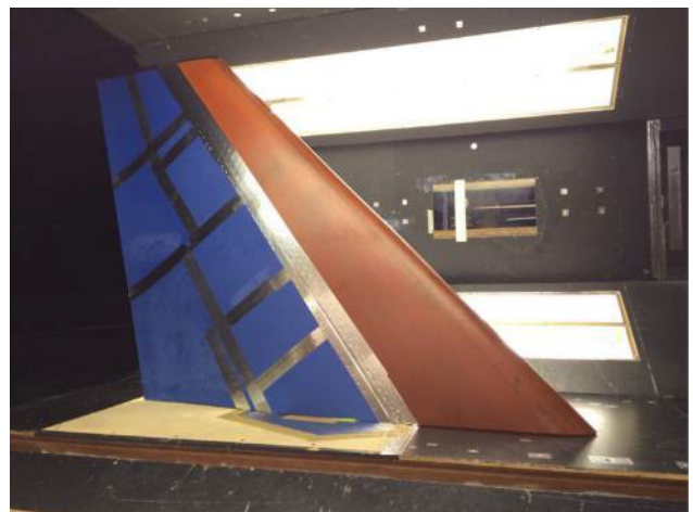
BILD 20: Einbau im Windkanal, Seitenansicht
