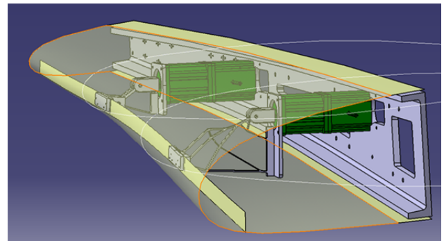
BILD 2: Konzept der Droopnose
