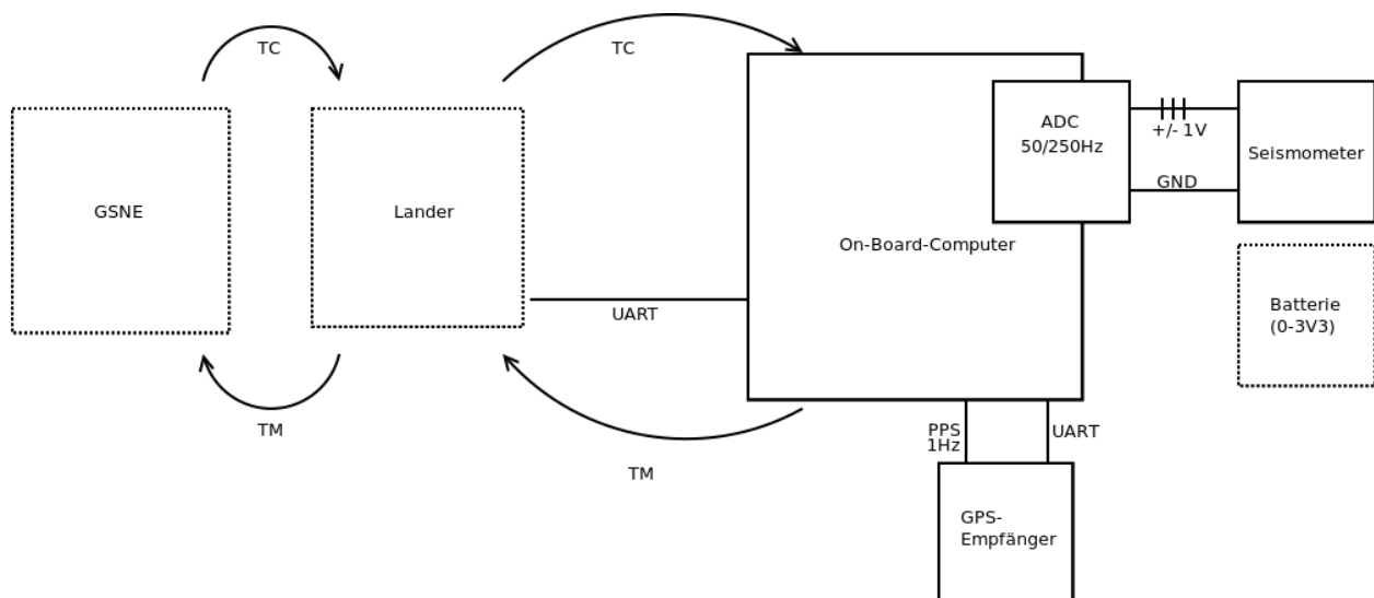
Abbildung 3.1: Allgemeiner Systemüberblick
