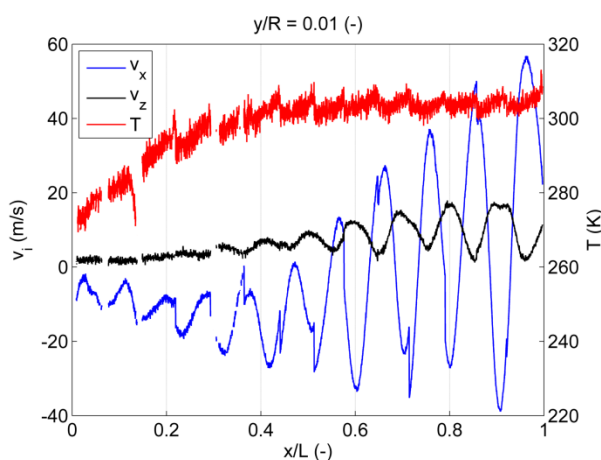
Abb. 5: Profile von v_x (blau), v_z (schwarz) und T (rot) bei y/R = 0,01
